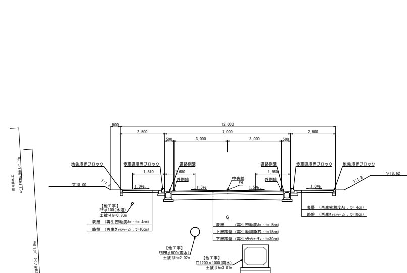
計画道路標準断面図
