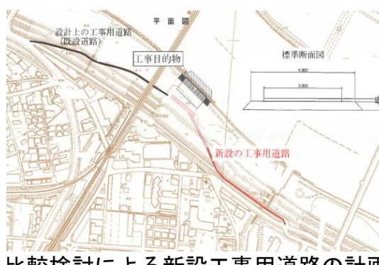
比較検討による新設工事用道路の計画
