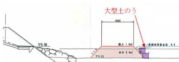
標準断面図
