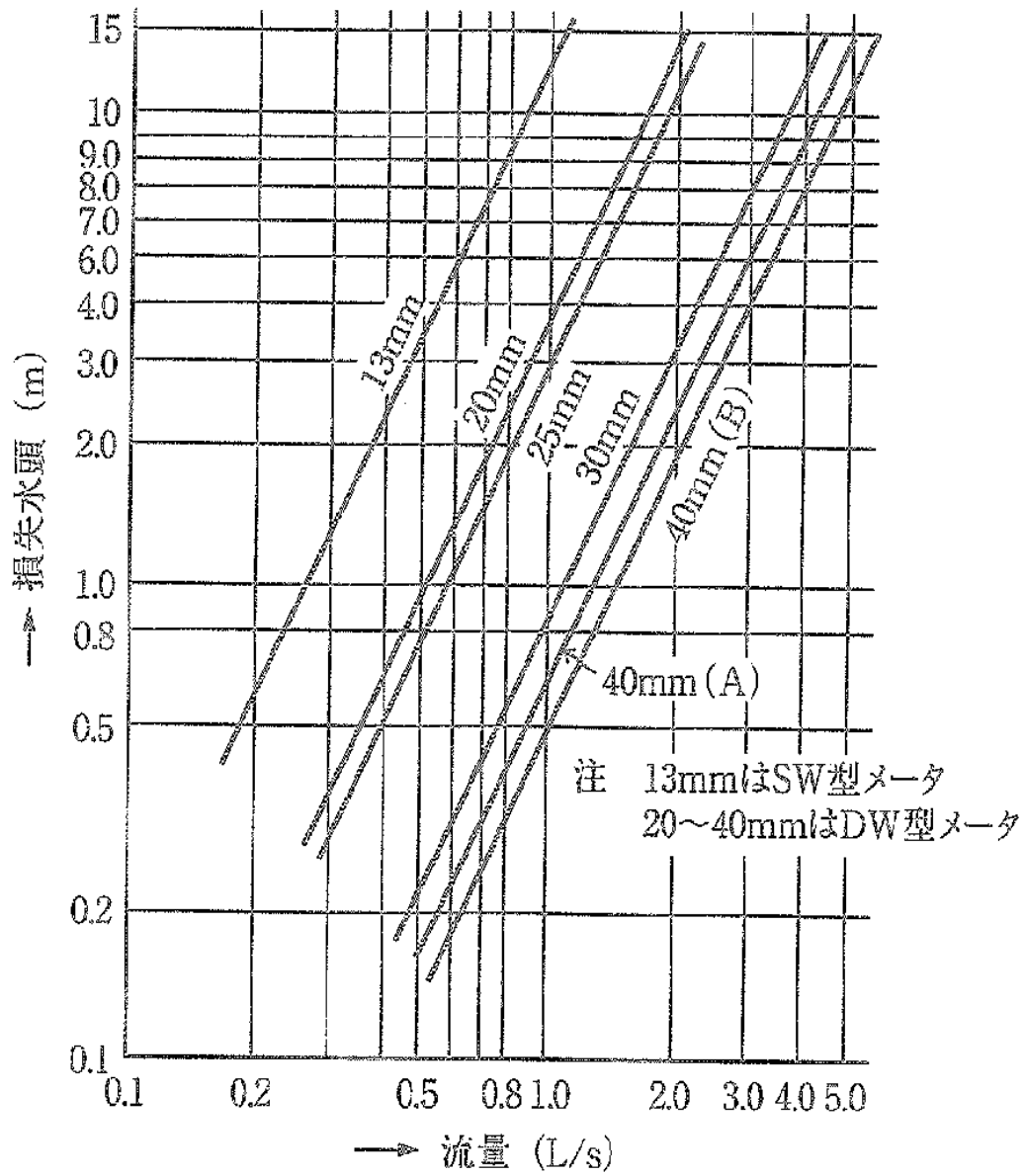
図 3.4.6 メーターの損失水頭例
