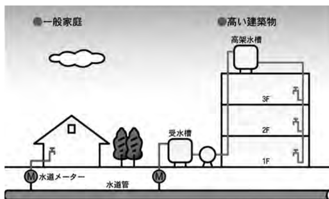
▲貯水槽のしくみ
